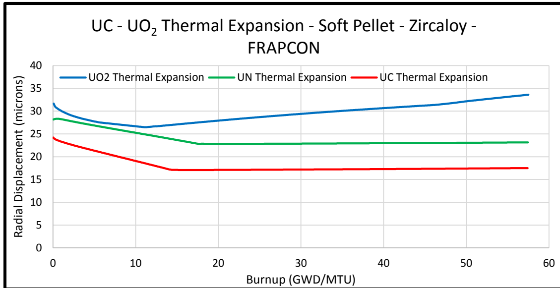
Figure 4.23: UC - UO_2 – UN Thermal Expansion Comparison
